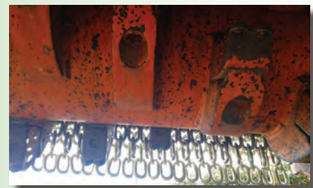
Forstrotor mit festen Werkzeugen
