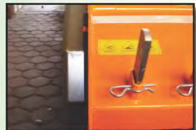
Holzaufnahmezinken (serienmäßig) in stabiler Tasche gehalten (herausnehmbar)
